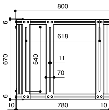
Sistema di fissaggio proiettore
