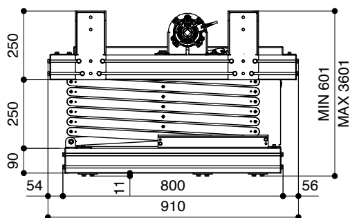
Vista laterale chiuso
