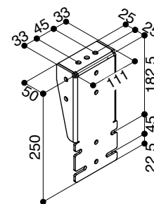
Staffa di ancoraggio a soffitto
